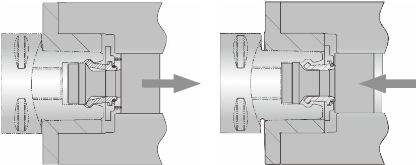
Принципиальная схема работы системы зажима инструмента стандарта PSC
