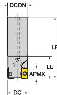
<C> Цилиндрическая фреза
