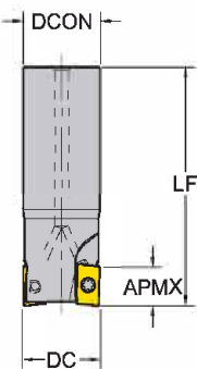
<C> Цилиндрическая фреза
