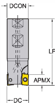
<W> Фреза с хвостовиком Weldon
