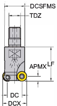
<M> Модульная фреза
