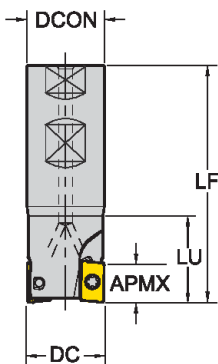
<W> с хвостовиком Weldon
