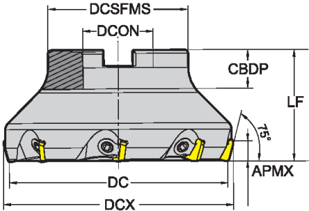
<S> Торцово-цилиндрическая фреза
