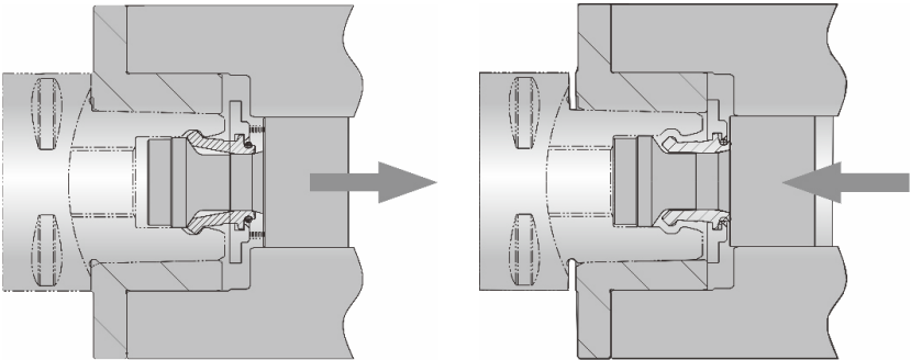
Принципиальная схема работы системы зажима инструмента стандарта PSC
