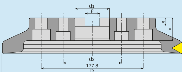
D TİP / D TYPE / D Тип
