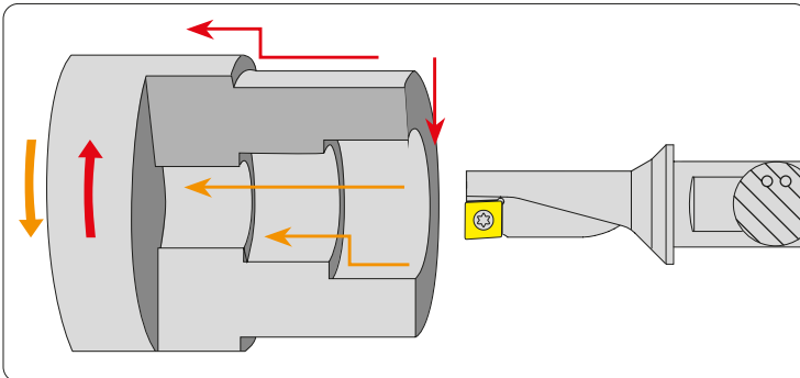
Delme Drilling Сверление
